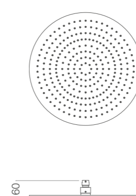
SK 004 ✓ Ø 400 mm ✓ G. ½" F
