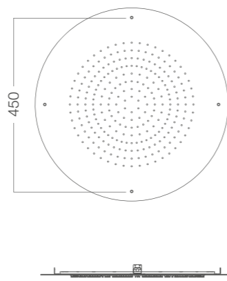
SK 016 ✓ Ø 500 mm ✓ G. ½" M
