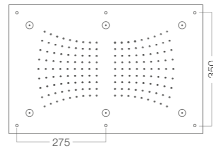
KI 221 / KI 261 ✓ L 600x400 mm ✓ G. 1/2" M
